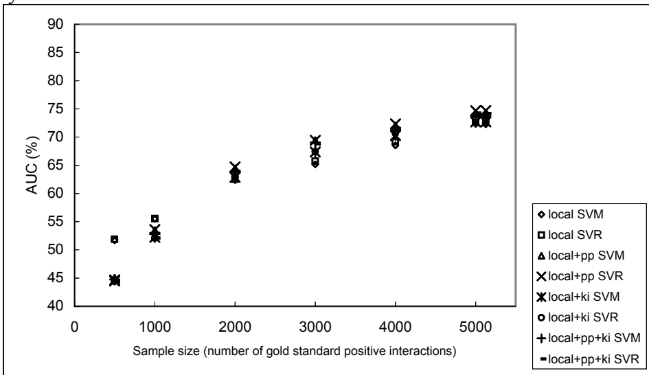
y2h-ito
